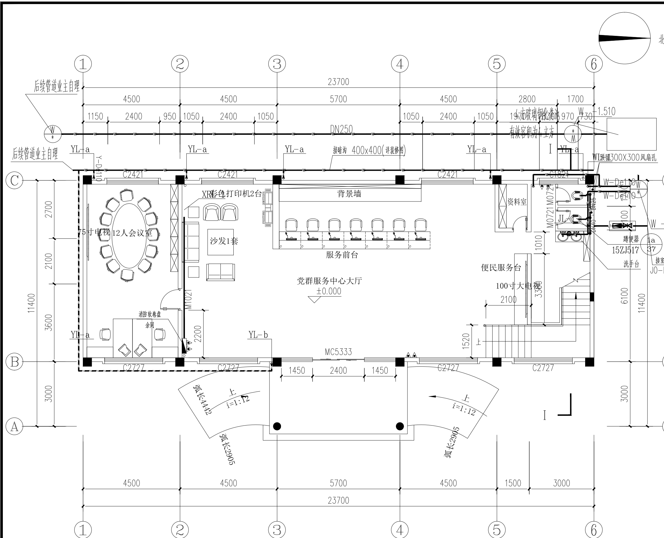
一层给排水平面图 1:100
