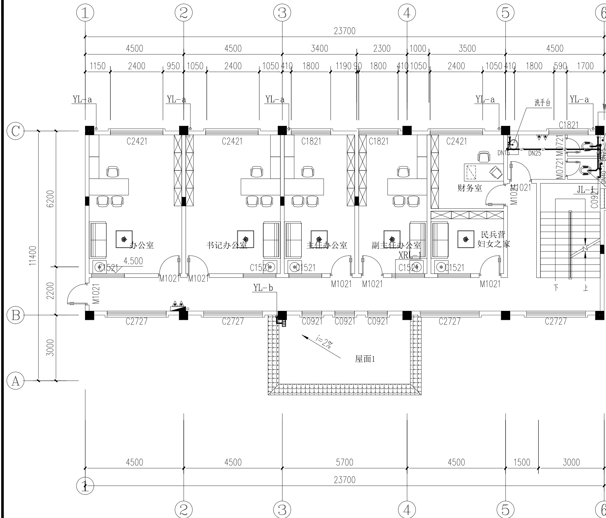
二层给排水平面图
