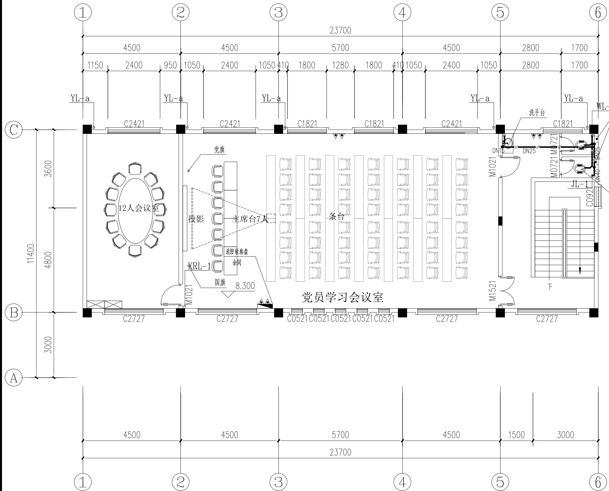
三层给排水平面图
