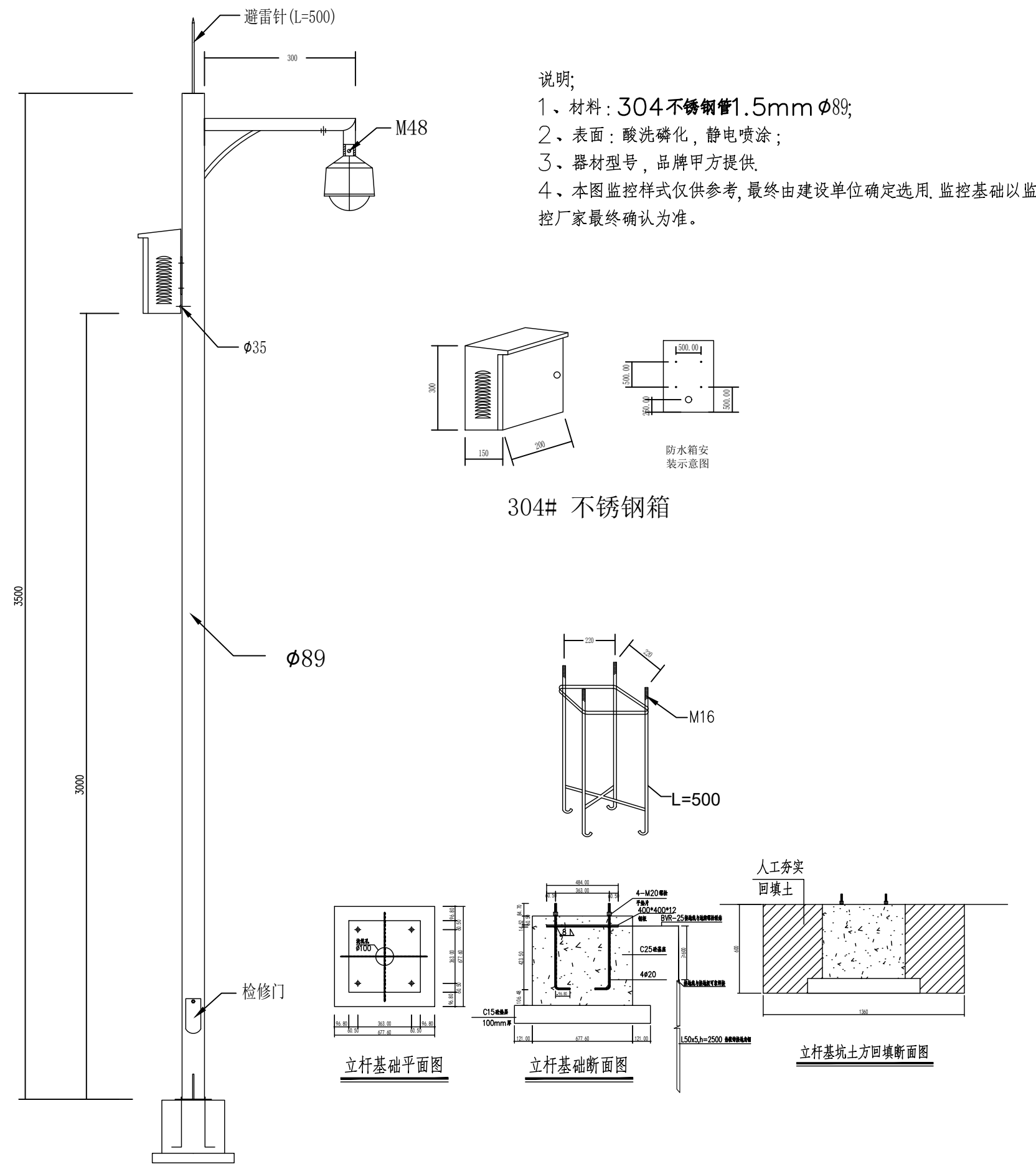
室外安防摄像机安装大样图
