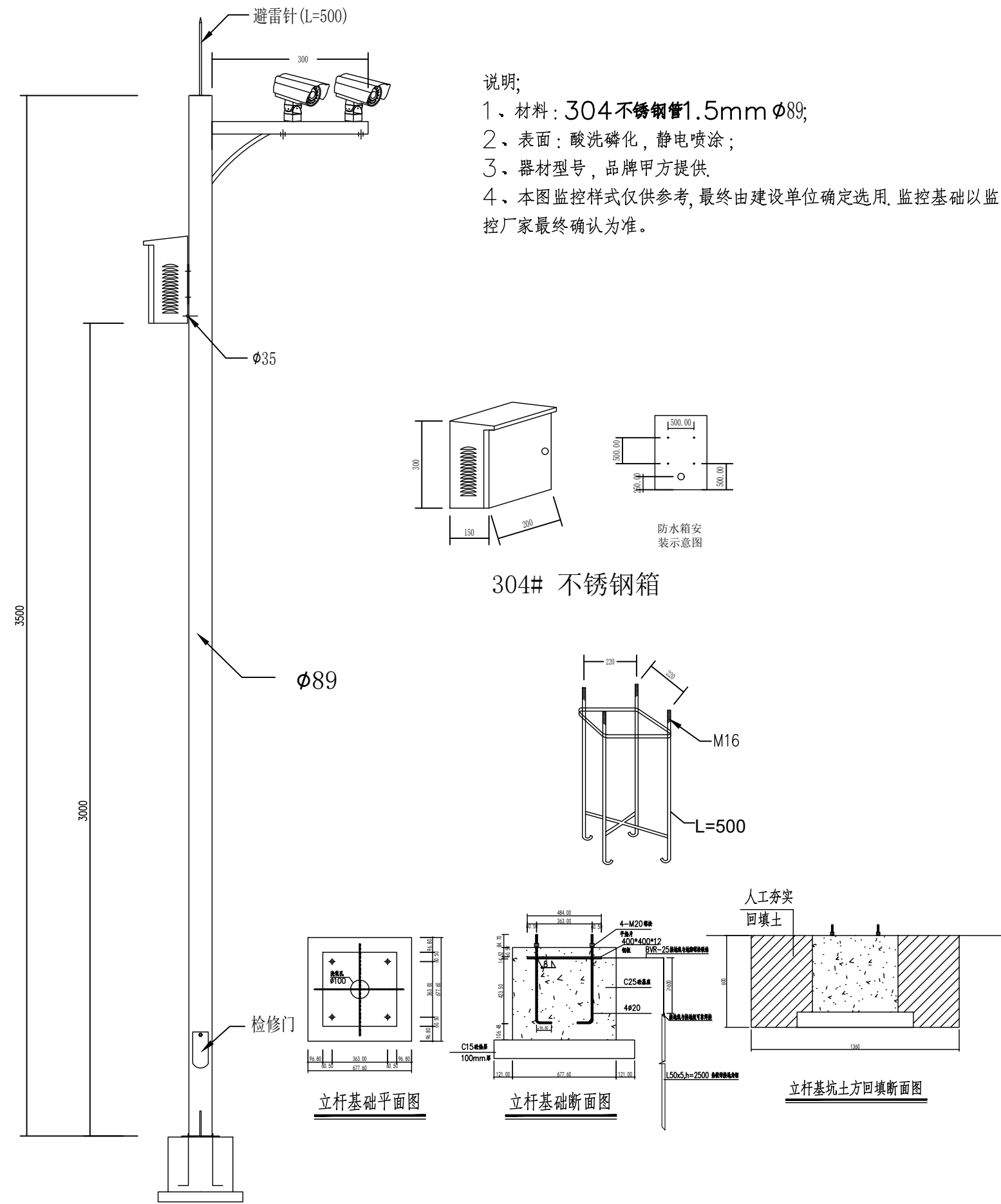
室外安防摄像机安装大样图
