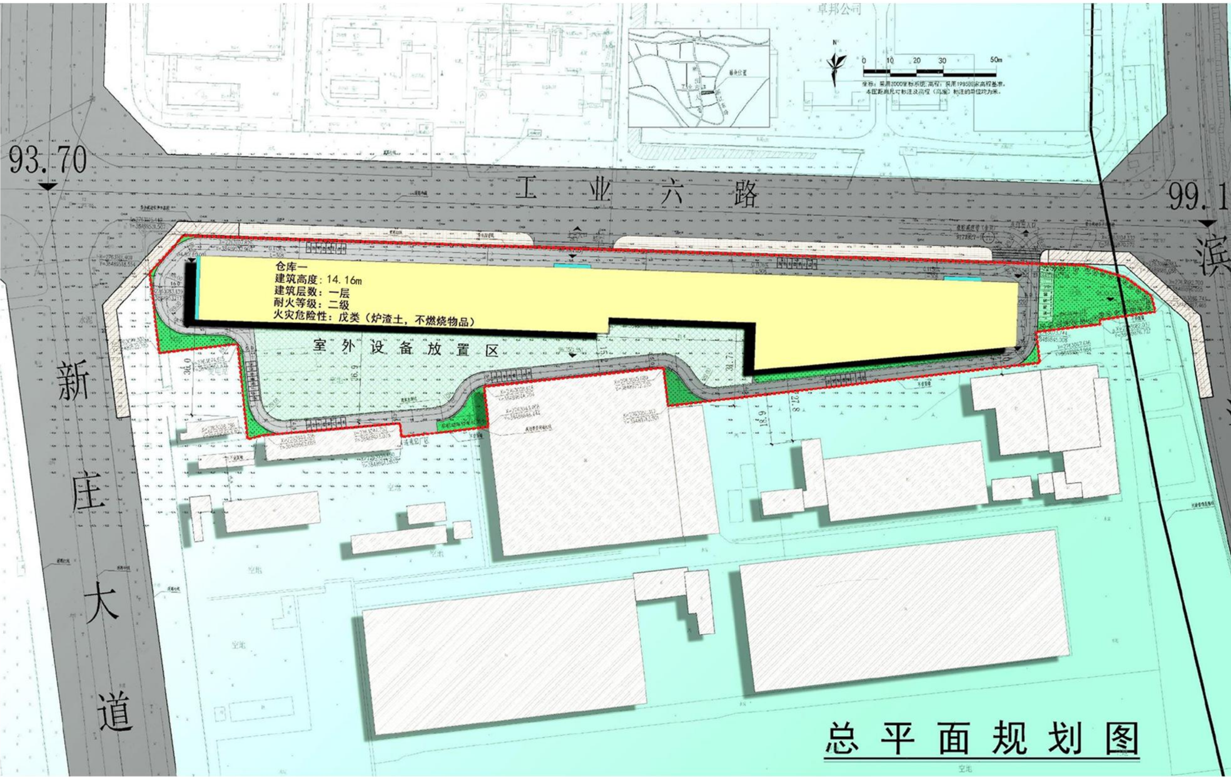
总平面图
