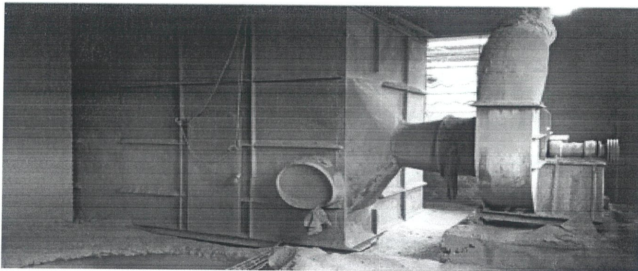
10 反吹袋式收尘机 (JH1-802)
