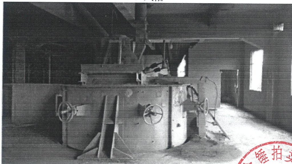
8选粉机（直径3.5M）
