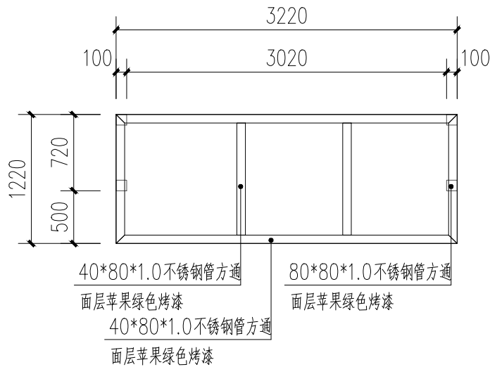
垃圾分类收集站屋架桁条平面图 1:50
