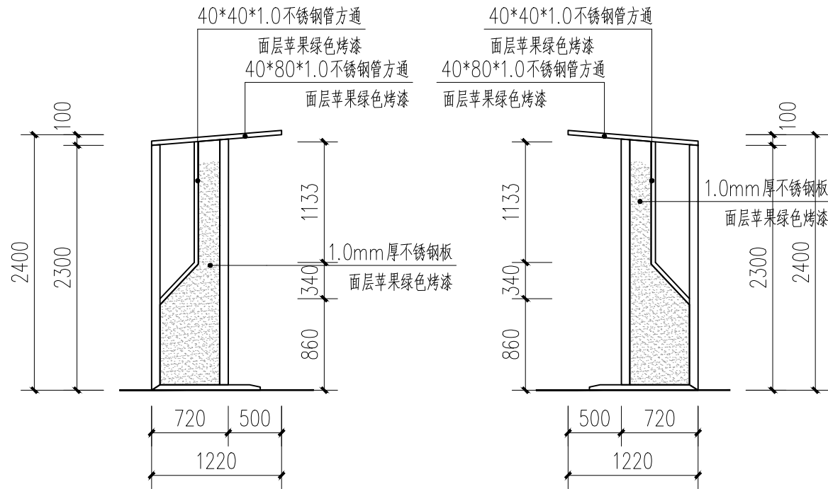
垃圾分类收集站左立面图 1:50
