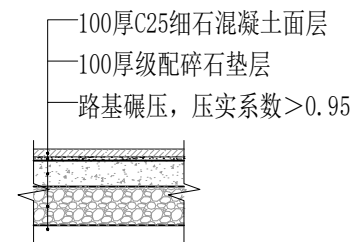
地面硬化做法 1:50
