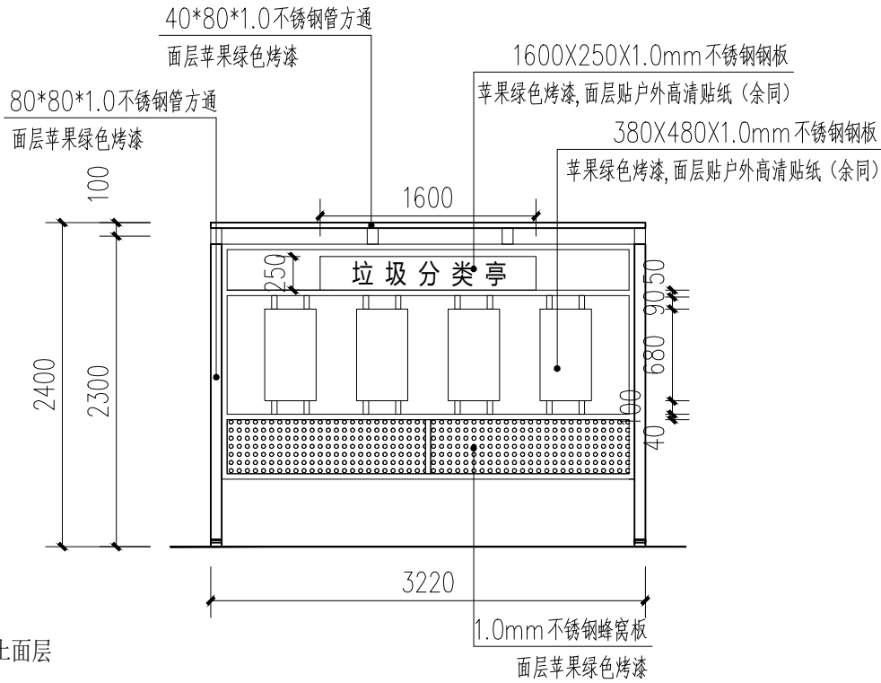
垃圾分类收集站立面图 1:50
