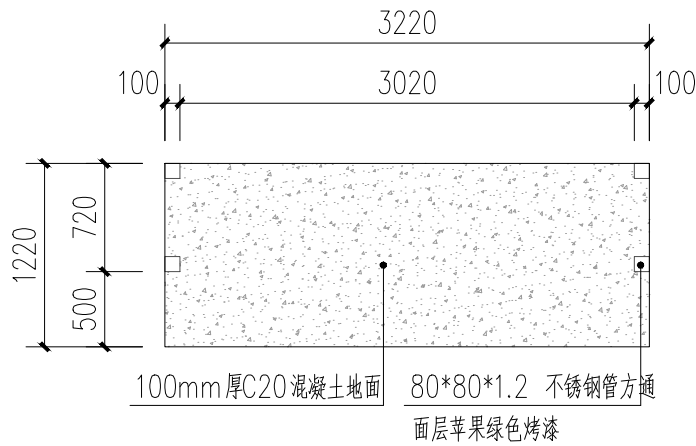
垃圾分类收集站地面平面图 1:50
