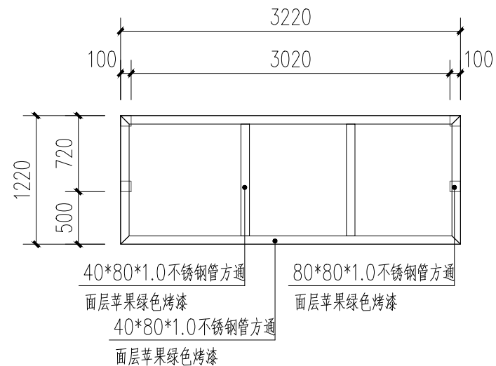
垃圾分类收集站屋架桁条平面图 1:50
