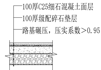
地面硬化做法 1:50
