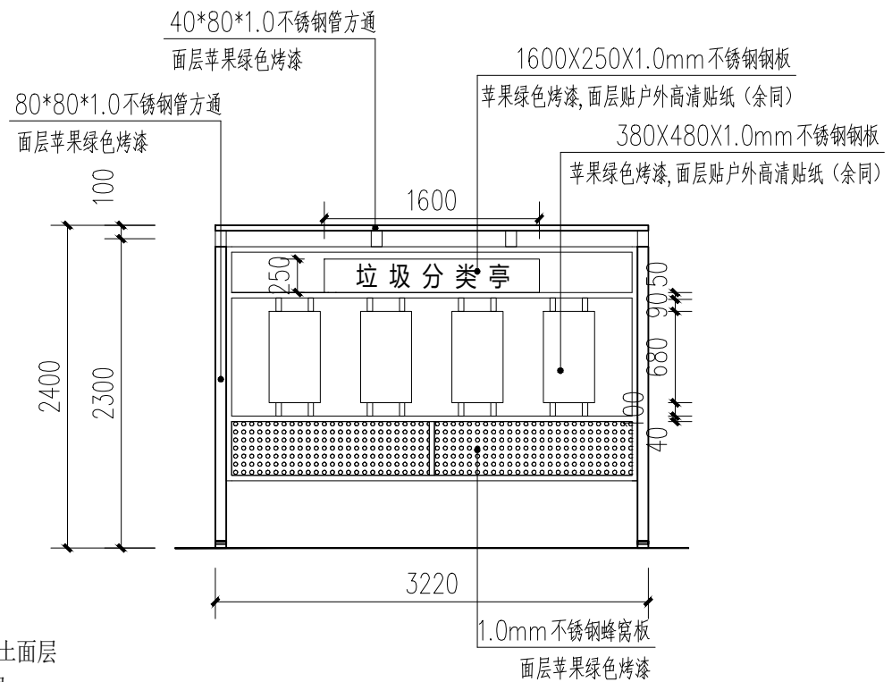
垃圾分类收集站立面图 1:50
