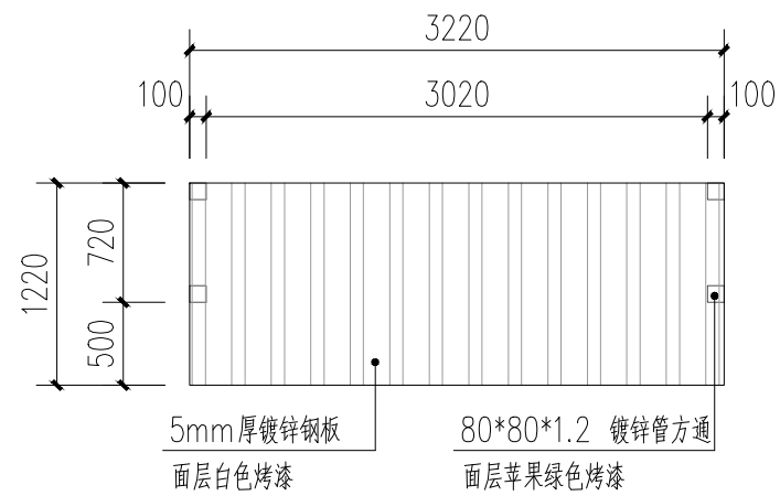
垃圾分类收集站顶平面图 1:50
