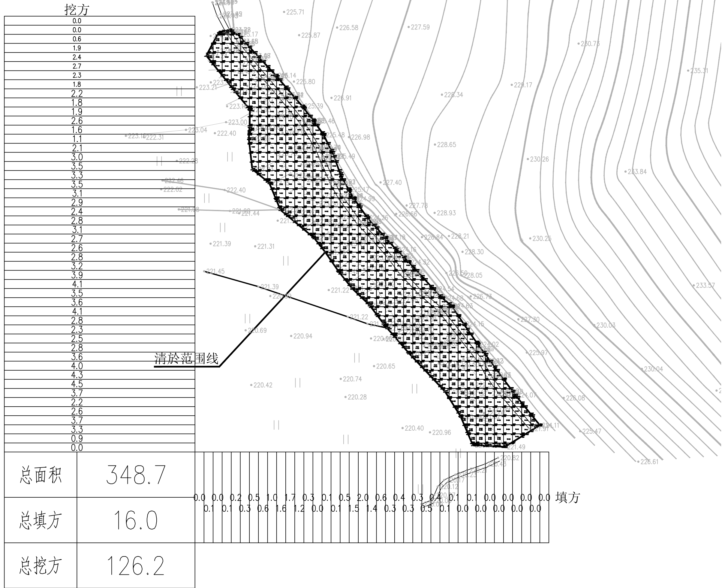
练屋村区域一清淤平面图 1:250
