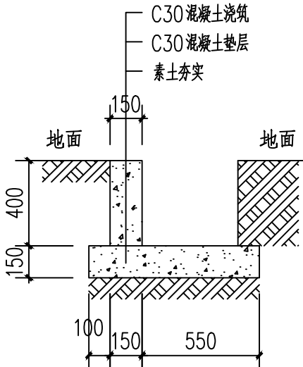
400单边水渠大样图 1:25
