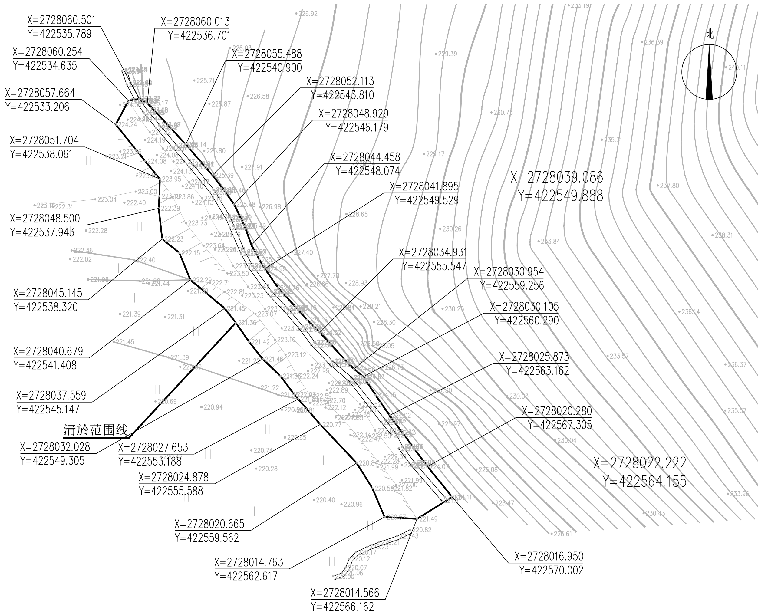
练屋村区域一平面图 1:250
