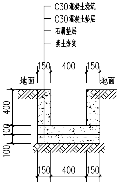
400*400三面光水渠大样图 1:25
