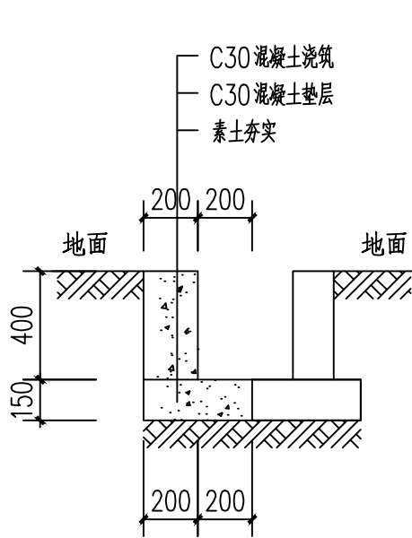
修复400*400三面光单边水渠大样图 1:25
