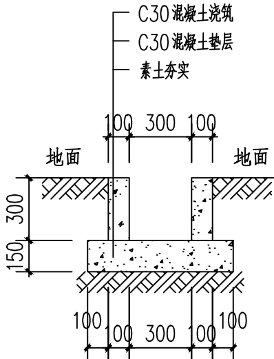
300*300三面光水渠一大样图 1:25
