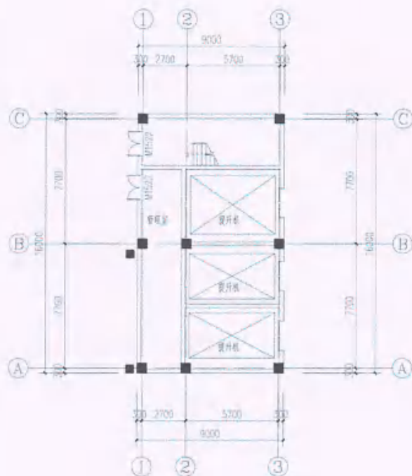
牛羊接收台一层平面图 1300
