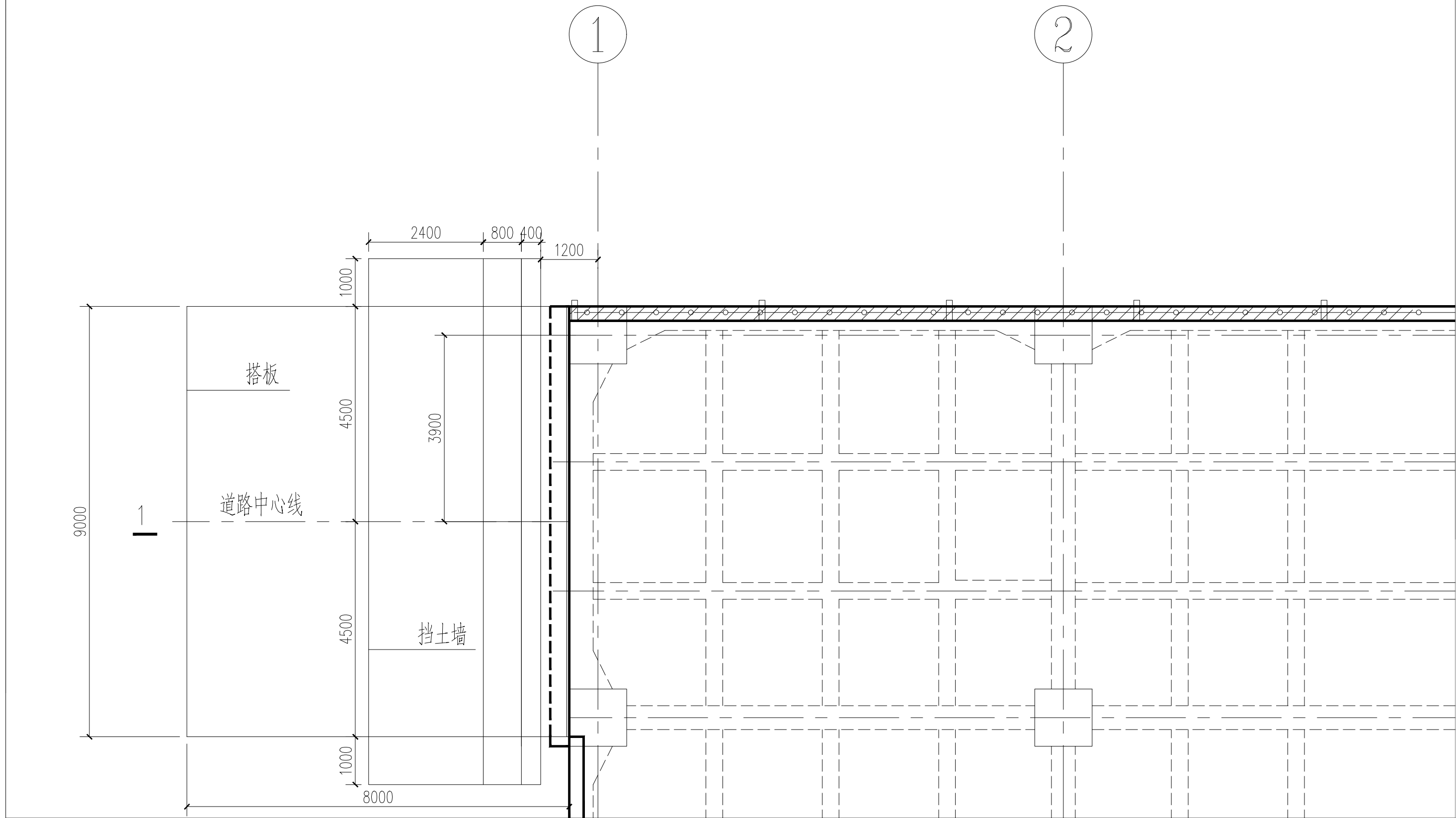
挡土墙及搭板平面布置图
