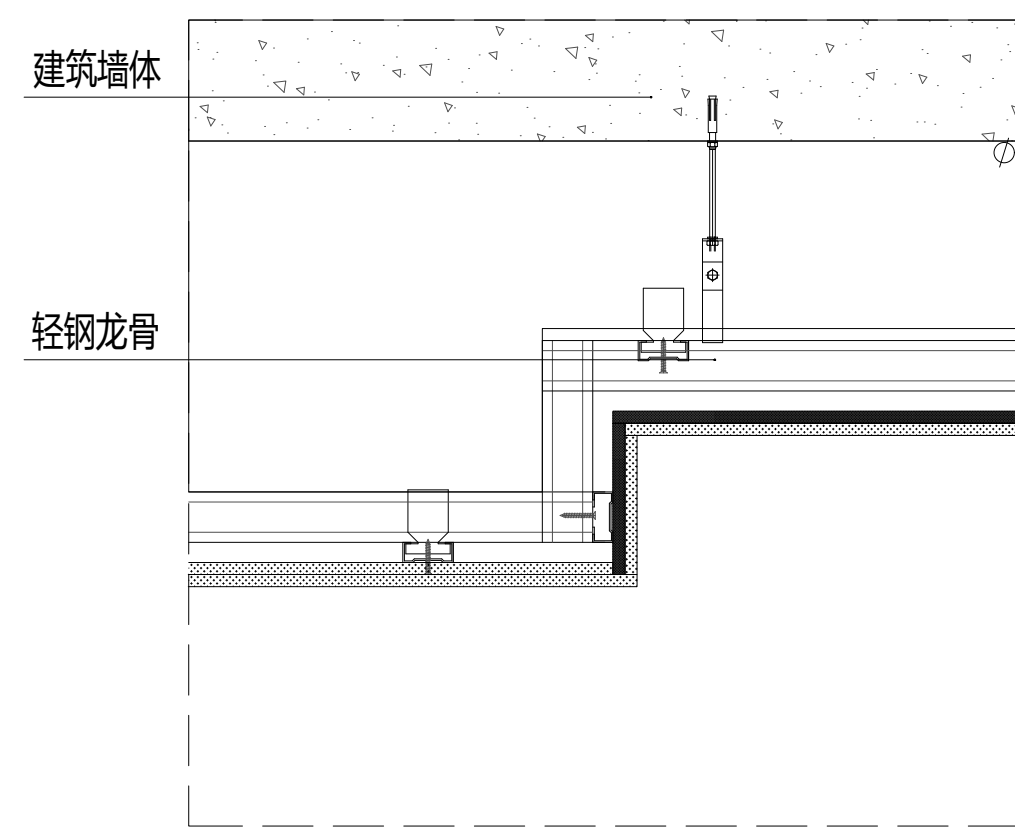
3 天花大样图 1:10
