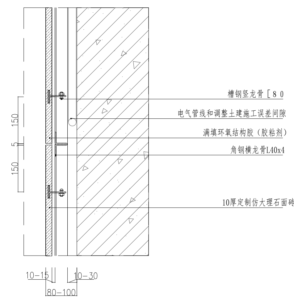
9 前台背景墙节点图2 1:10
