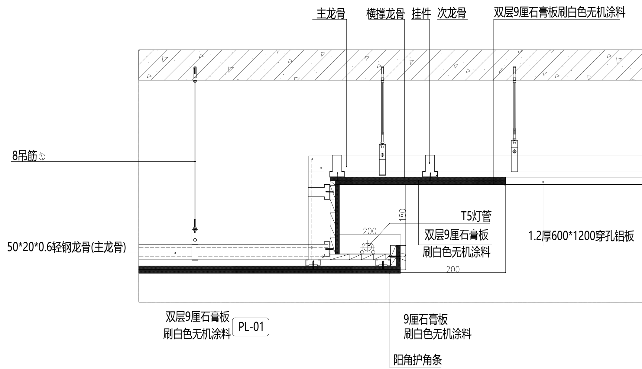
2 天花大样图 1:10
