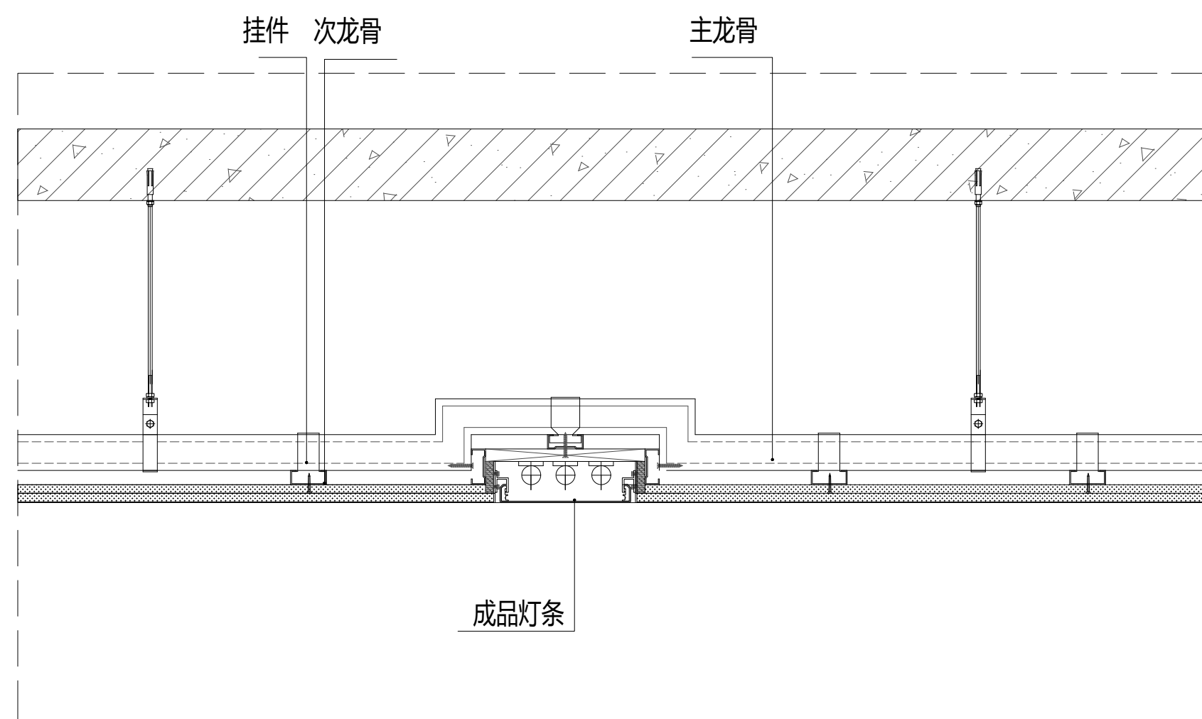
5 天花大样图 1:10
