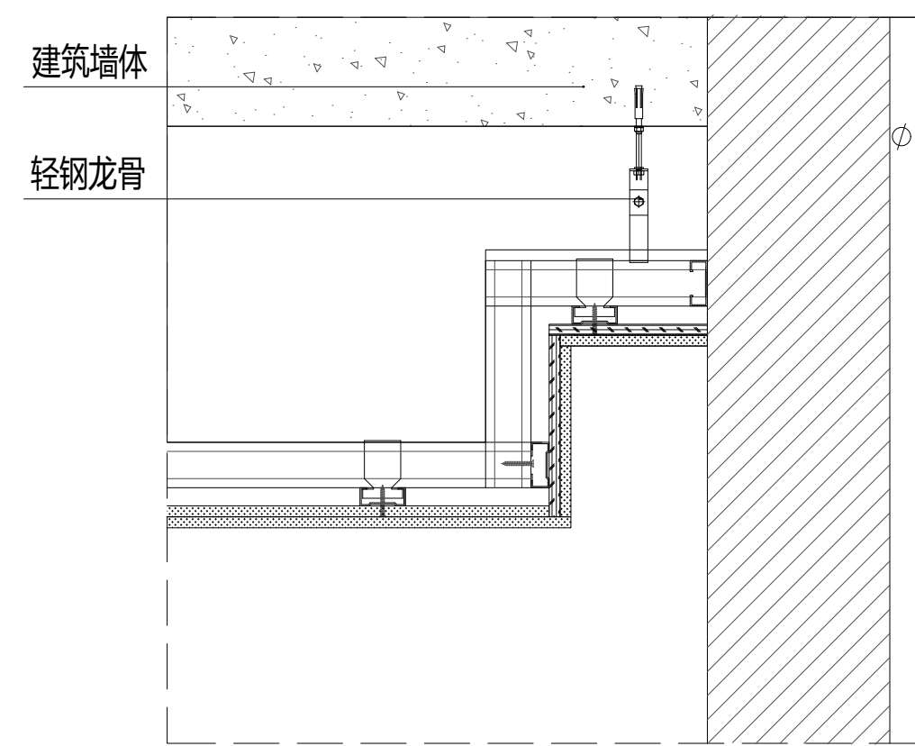
7 投影盒天花节点图 1:10
