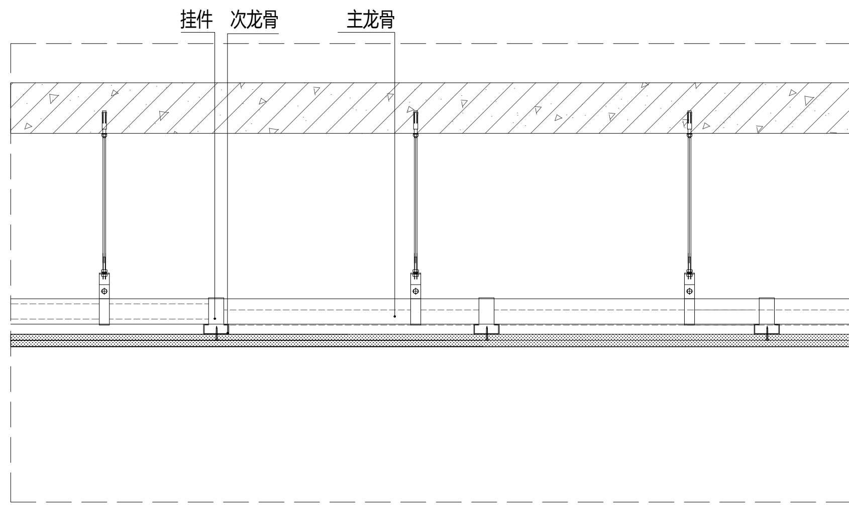
4 天花大样图 1:10
