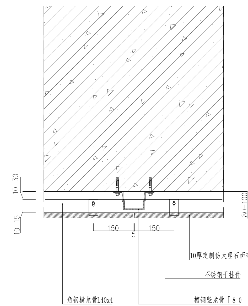
8 前台背景墙节点图1 1:10
