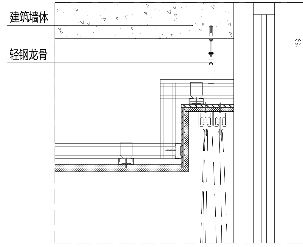
1 天花大样图 1:10
