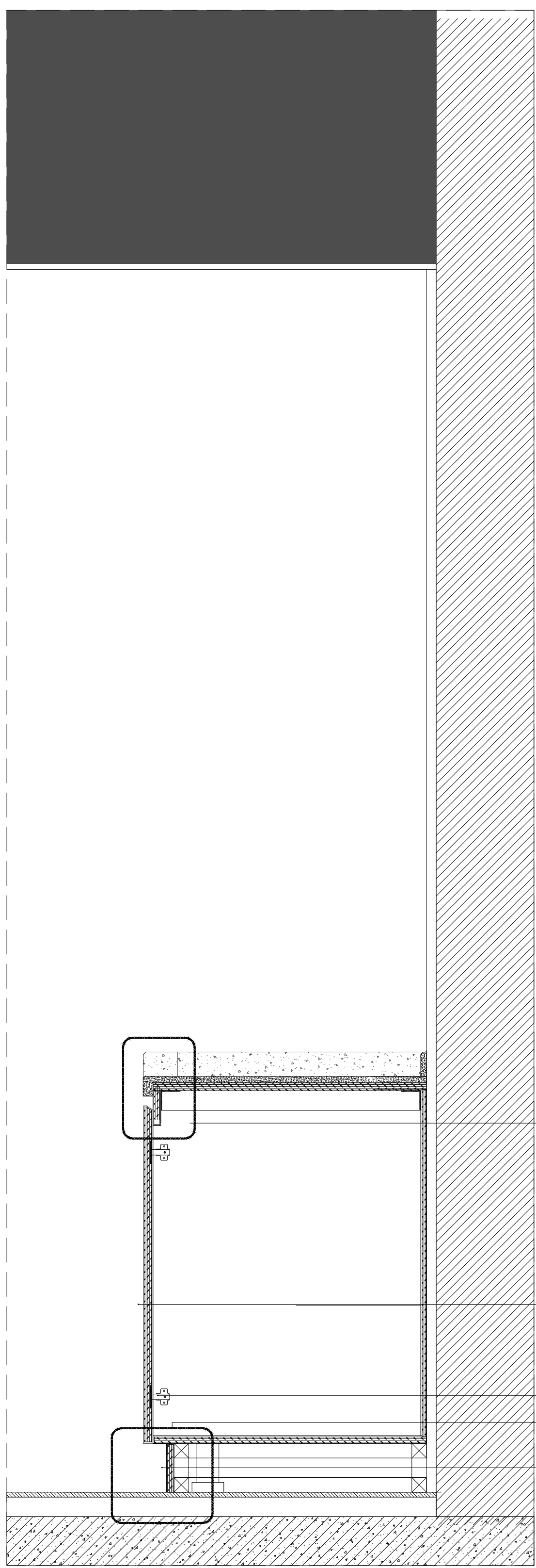
4 天花大样图 1:10
