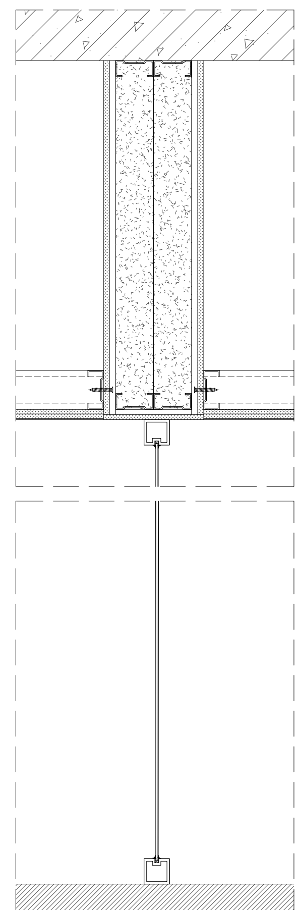
9 玻璃隔墙大样图 1:10
