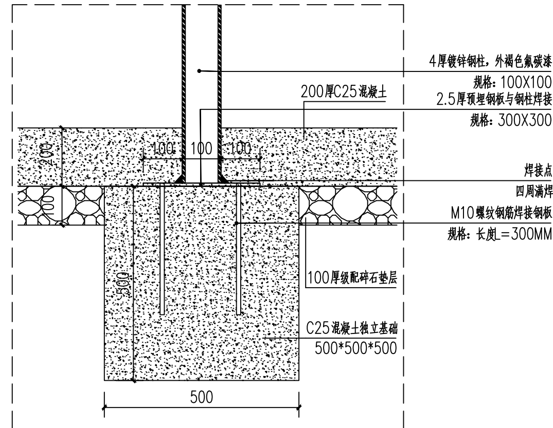
2 垃圾棚剖面图二 1:20
