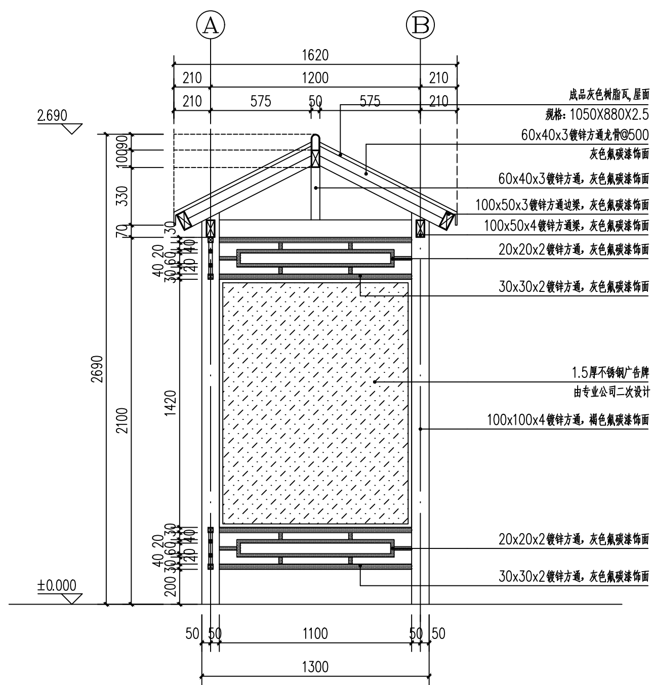
2 垃圾棚剖面图二 1:20
