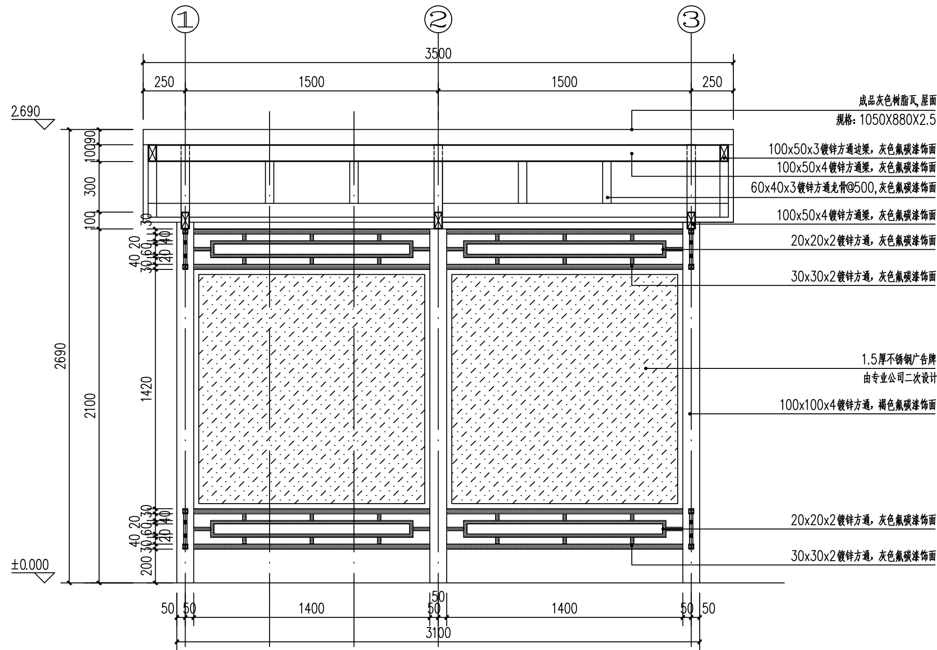
1 垃圾棚剖面图一 1:20
