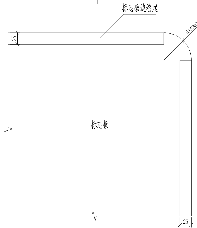
板面构造图 1:1
