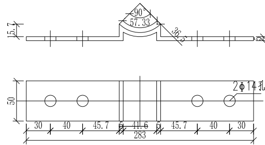
立柱底衬大样图
