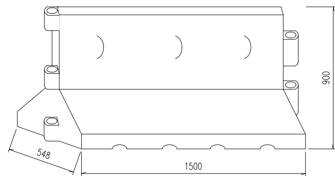
活动式防撞墙 1: 20
