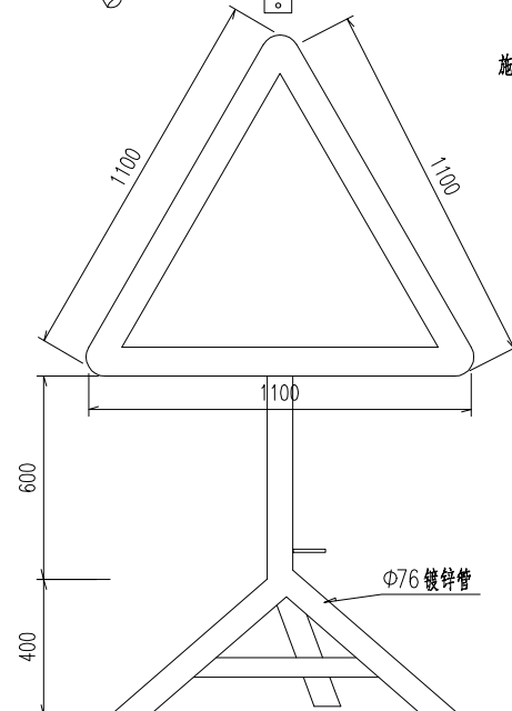
限速标志 1: 20
