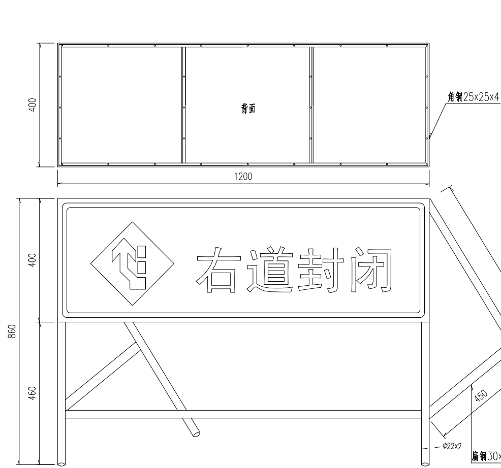
施工标志 1: 10
