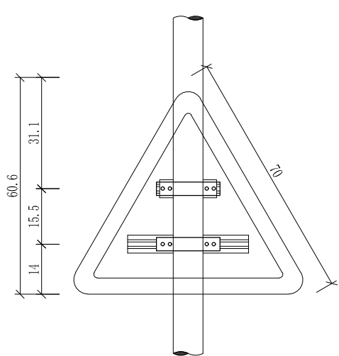
标志板背面连接图 1:15
