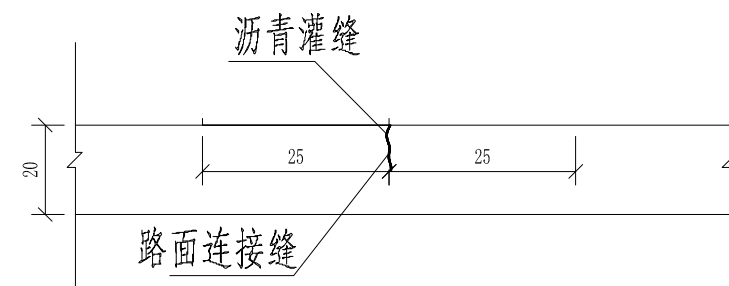
截面B-B
