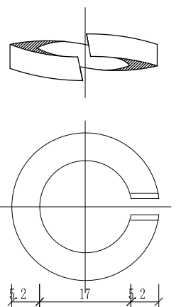
弹簧垫片大样图 1:1
