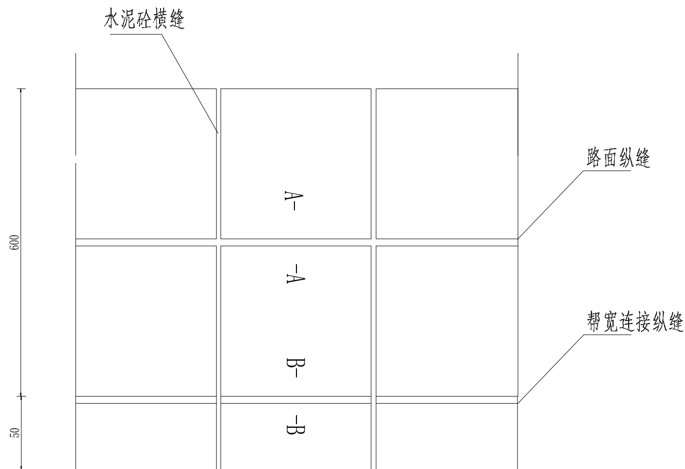
原路面帮宽接缝平面布置图
