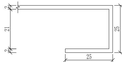
卷边大样图
