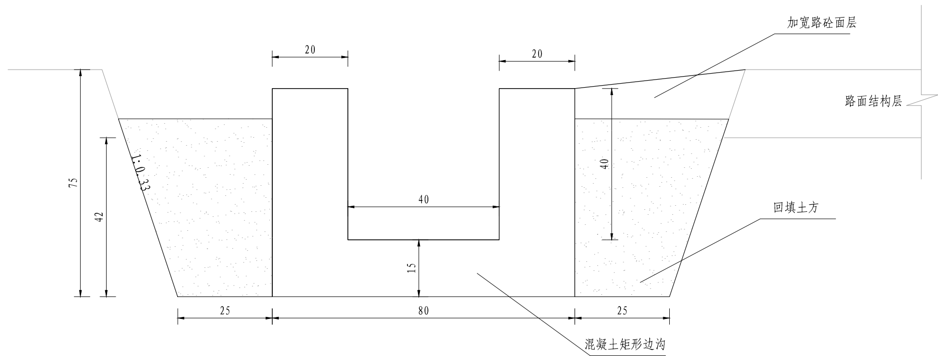
矩形边沟大样图
