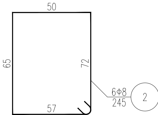
基础钢筋大样 1:15
