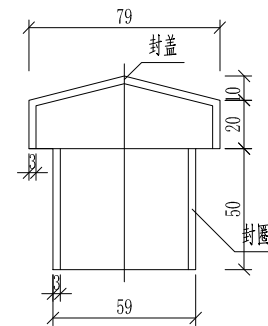
柱帽大样图
