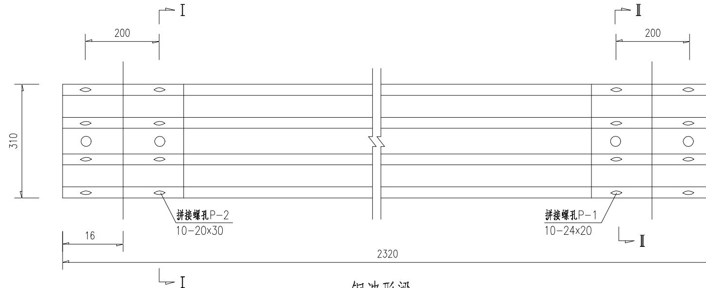
钢波形梁 1:10
