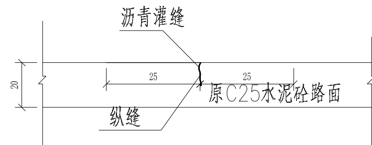
截面A-A
