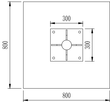
I—I 1:20
