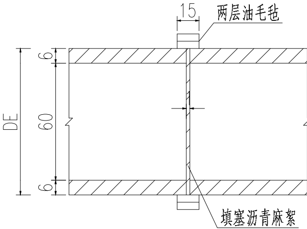
管节接头
