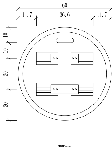
标志板背面连接图 1:15
