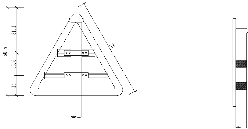
标志板背面连接图
