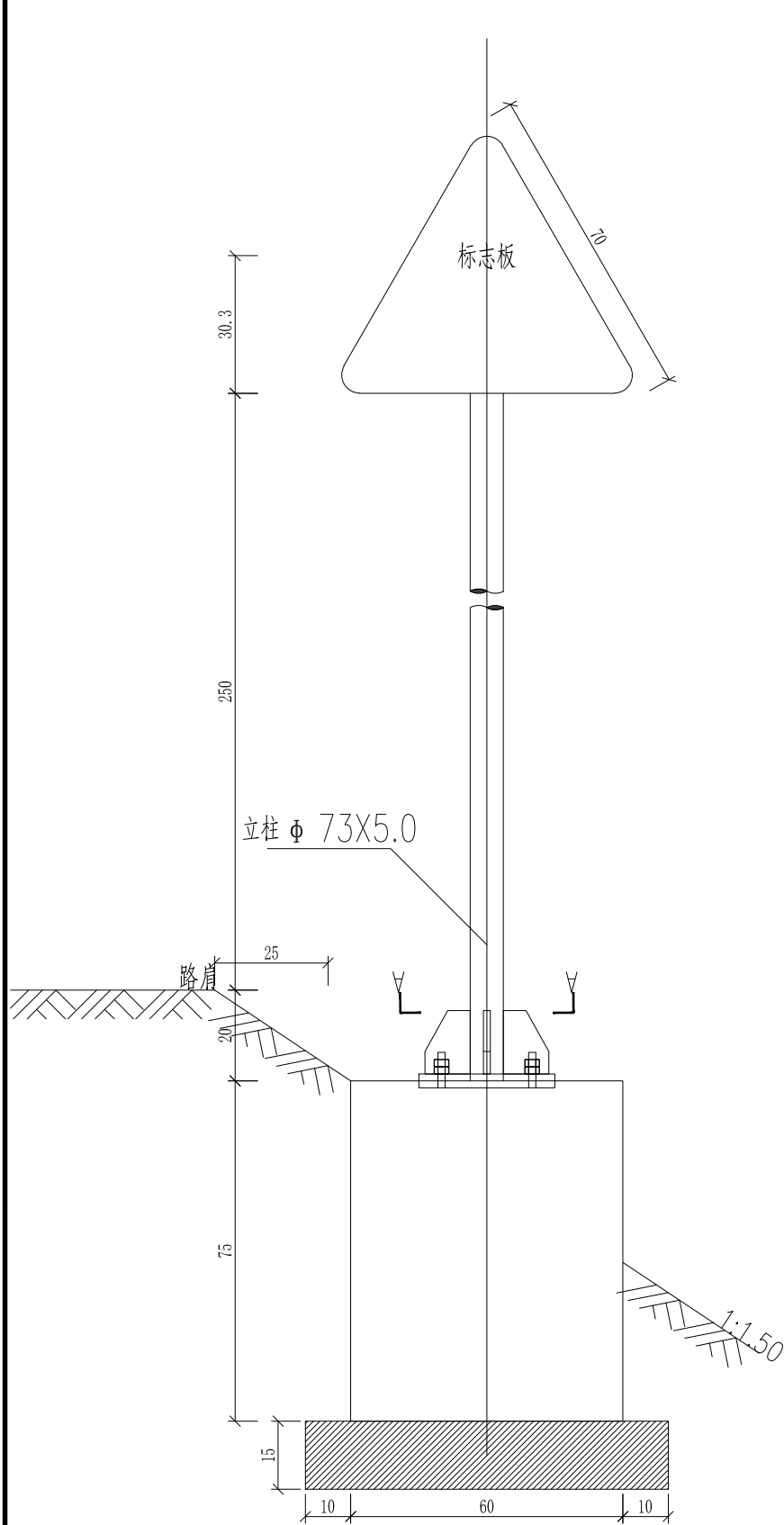
标志立面图
