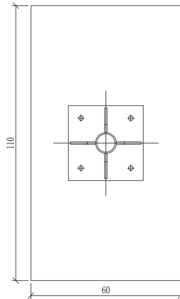
A-A剖面 1:15
