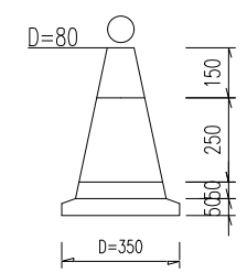
配有施工警告灯的锥形交通路标 1: 20
