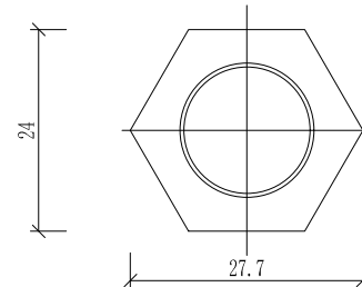
螺母大样图 1:1
