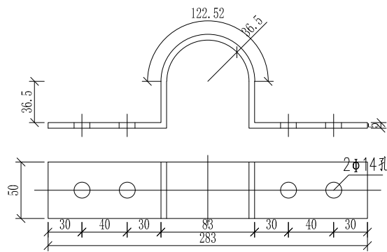
抱箍大样图
