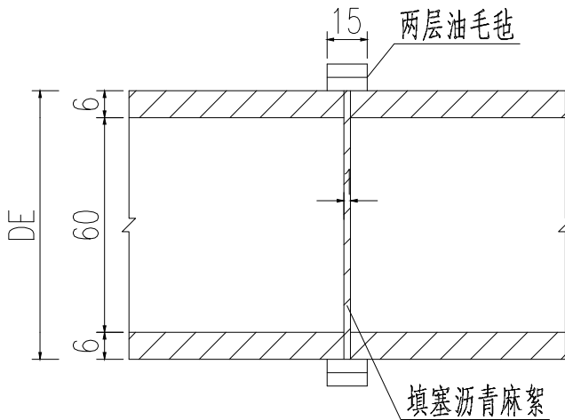
管节接头 1:20
