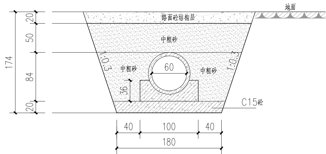
水泥涵管大样 1:50
