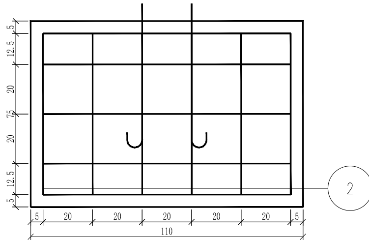
侧面图 1:15
