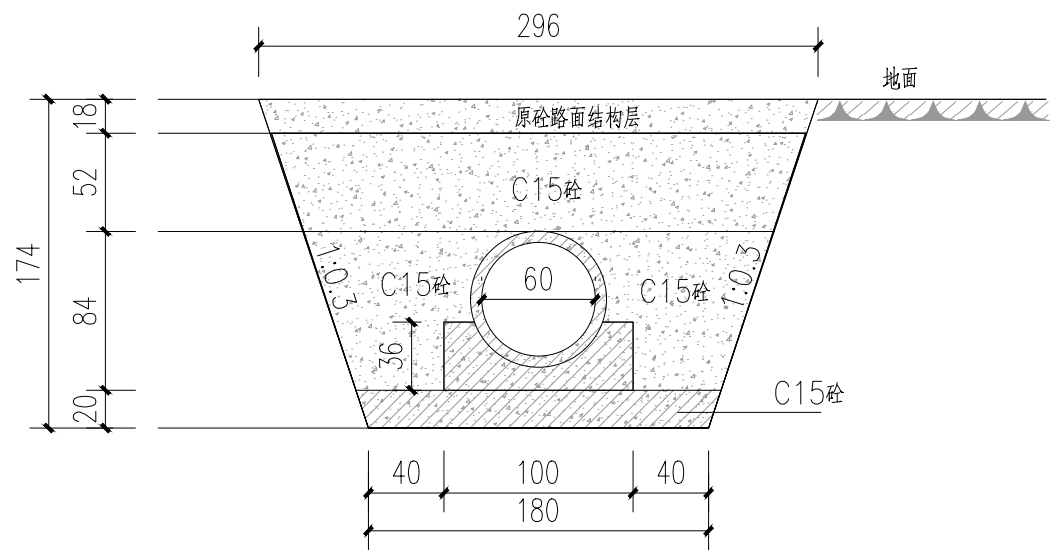
过路水泥涵管大样 适用过路砼管部位
