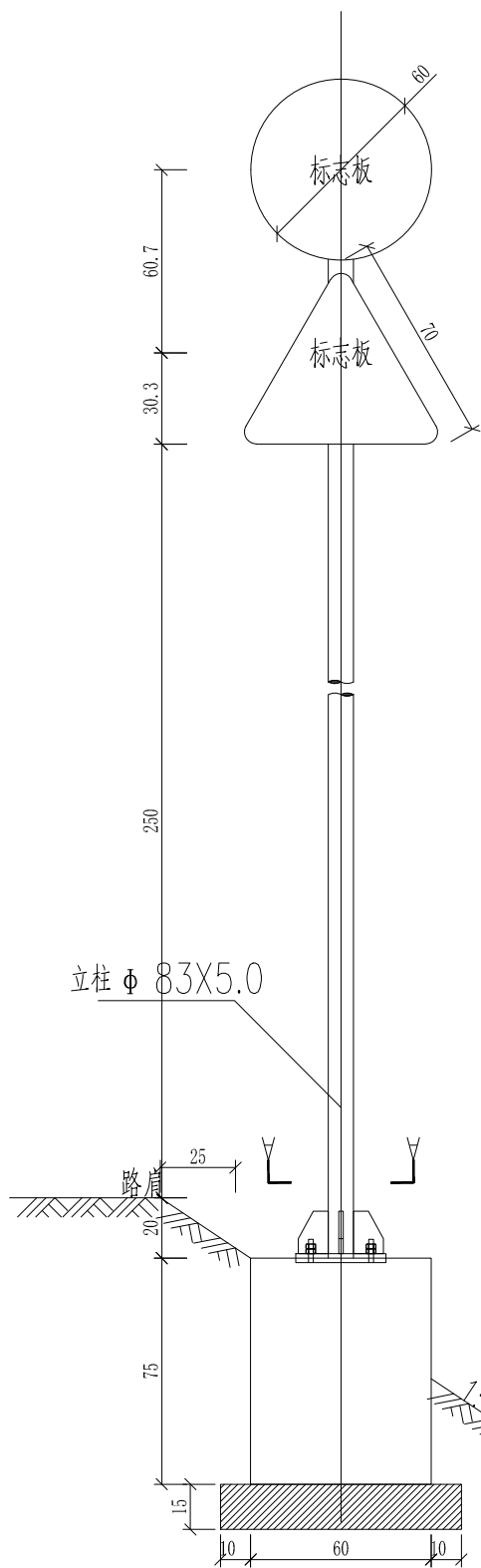
标志立面图 1:25
