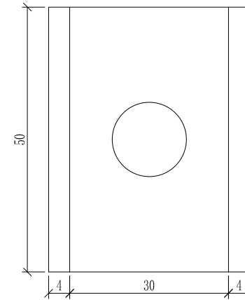
滑块大样图 1:1
