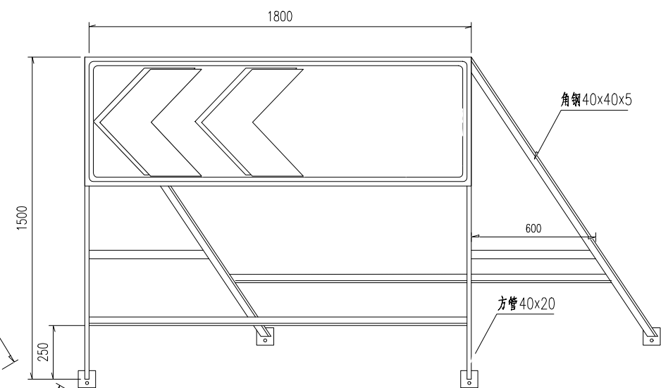
施工标志 1: 20
