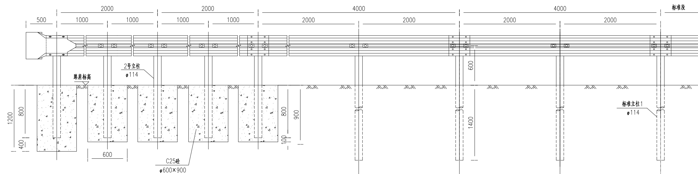
护栏上游端头平面图
