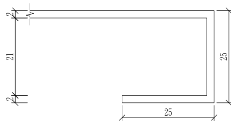
卷边大样图 1:1
