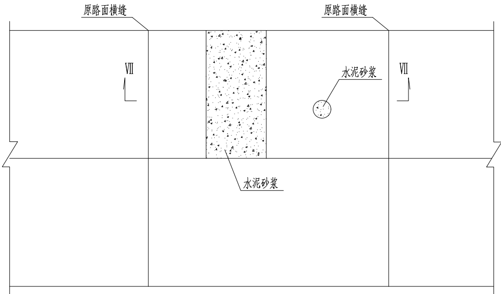
病害处理平面图
