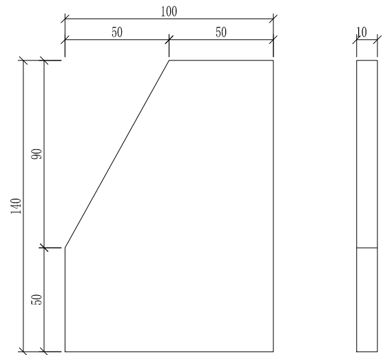
肋板大样图 1:2
