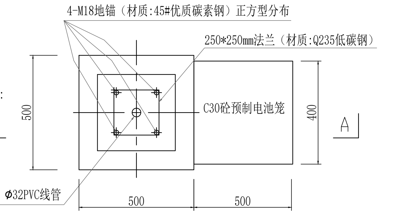
基础(JC-1)平面图
