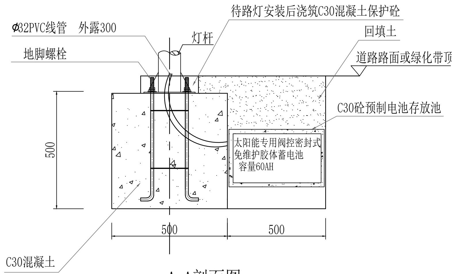
A-A剖面图
